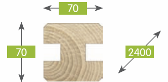
192601A001AABZ80A1 744 Krawędziak H21 70x70x2400 SF Post H21 70x70x2400 PC Poteau H21 70x70x2400 RC Kantholz H21 70x70x2400 geh gefast
