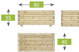
240106B023OMBZ09A1 957 Kwietnik 80x35x40 ram R35x45 Flower box 80x35x40 F35x45 Bac 80x35x40 C35x45 Pflanzkasten 80x35x40 R35x45
