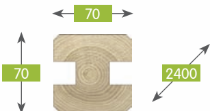
192601B001AABZ80A1 746 Krawędziak H21 70x70x2400 SF Post H21 70x70x2400 PC Poteau H21 70x70x2400 RC Kantholz H21 70x70x2400 geh gefast
