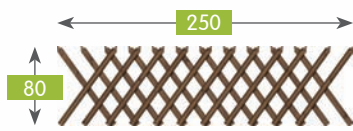
1203 Myśliwski tocz 250x80 ostrz 55 Hunting fence turned 250x80 pointed 55 Clôture croisée ronde 250x80 app 55 Jägerzaun gek 250x80 gesp 55
