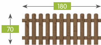
1182 Sztachetowy 180x70 D15x90-11 R25x70 trapez BF Pale fence 180x70 P15x90-11 trapez nch Clôture stackette 180x70 S15x90 trapeze Staketenzaun 180x70 S15x90-11 Trapez of
