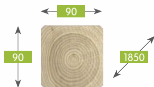
190101A032AABZ55A1 601 Krawędziak 90x90x1850 SF Post 90x90x1850 PC Poteau 90x90x1850 RC Kantholz 90x90x1850 geh gefast
