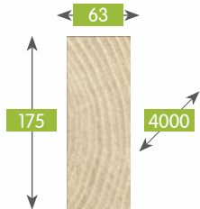
200101A021AACZ20A1 758 Łata 63x175x4000 po pile Lath 63x175x4000 after saw Lambourde 63x175x4000 brutte Konstruktionsholz 63x175x4000 gesägt
