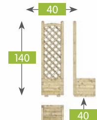
240108A004MSCZ20A1 964 Kwietnik 40x140x40 ram KR ł R30x60 Flower box 40x140x40 tr arch F30x60 Bac à fleur 40x140x40 treillis arc C30x60 Pflanzkasten 40x140x40 Gitt B R30x60
