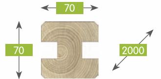
192601A002AABZ80A1 745 Krawędziak H21 70x70x2000 SF Post H21 70x70x2000 PC Poteau 70x70x2000 RC Kantholz H21 70x70x2000 geh gefast
