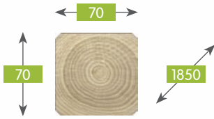
620 190101B011AABZ80A1 Krawędziak 70x70x1850 SF Post 70x70x1850 PC Poteau 70x70x1850 RC Kantholz 70x70x1850 geh gefast
