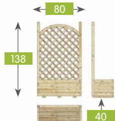
240108A003OSCZ12A1 963 Kwietnik 80x138x40 ram KR ł R30x60 Flower box 80x138x40 tr arch F30x60 Bac à fleur 80x138x40 treillis arc C30x60 Pflanzkasten 80x138x40 Gitt B R30x60
