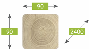
626 190102A005AACZ52A1 Krawędziak 90x90x2400 SR Post 90x90x2400 PR Poteau 90x90x2400 RR Kantholz 90x90x2400 geh R
