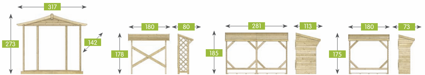
1089 261400B001OMBZ01A1 Pawilon pół-6-kątny 317x273x142 PD Pavillon half hexag 317x273x142 FL Pavillon demi hexag 317x273x142 L Pavillon halb - sechseckig 317x273x142 Fussb
