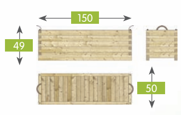
240206B008OMBZ04A1 968 Kwietnik 150x49x50 ram wr R45x90 Flower box 150x49x50 F45x90 Bac 150x49x50 C45x90 Pflanzkasten 150x49x50 R45x90
