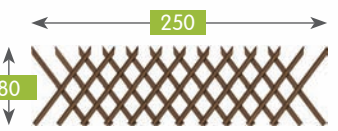
1206 Myśliwski str 250x80 zac 23x46 Hunting fence planed 250x80 cut 23x46 Clôture croisée rb 250x80 ent 23x46 Jägerzaun geh 250x80 angesch 23x46
