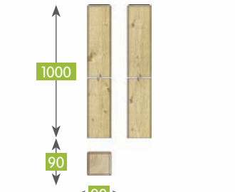
192301A003AABZ48A1 741 Krawędziak łeb4F 90x90x1000 SF Post head 4CH 90x90x1000 PC Poteau 90x90x1000 RC łęte 4CH Kantholz Kopf4F 90x90x1000 geh gefast
