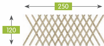
364 Myśliwski tocz 250x120 ostrz 46 Hunting fence turned 250x120 pointed 46 Clôture croisée ronde 250x120 app 46 Jägerzaun gek 250x120 gesp 46
