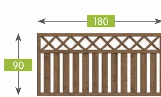
1176 Deskowy rama krzyż X 180x90 R45x45 D16x88 Plank fence cross X 180x90 F45x45 P16x88 Panneau planche cadre croix X 180x90 C45x45 Bretterzaun Kreuz X 180x90 R45x45 B16x88
