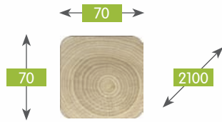
623 190102A002AACZ80A1 Krawędziak 70x70x2100 SR Post 70x70x2100 PR Poteau 70x70x2100 RR Kantholz 70x70x2100 geh R
