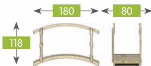
1141 Mostek 180x118x80 poręczce Bridge 180x118x80 rails Pont 2 rampes 180x118x80 Brücke 180x118x80 Geländer
