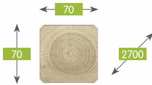
616 190101A067AACZ48A1 Krawędziak 70x70x2700 SF Post 70x70x2700 PC Poteau 70x70x2700 RC Kantholz 70x70x2700 geh gefast
