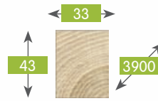
200101A010AACZ150A 750 Łata 43x33x3900 po pile Lath 43x33x3900 after saw Lambourde 43x33x3900 brutte Konstruktionsholz 43x33x3900 gesägt
